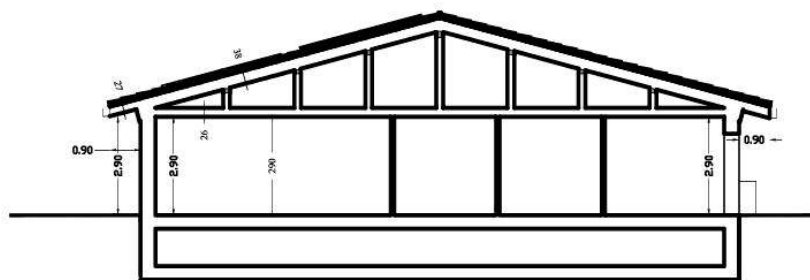
SEZIONE
